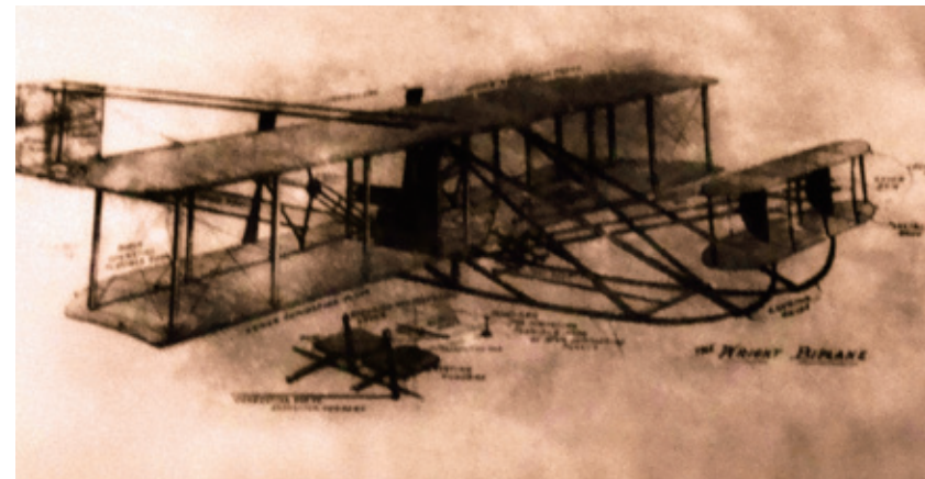
图 2: 莱特双翼飞机结构图。冯如 1909 年设计、制造飞机的蓝本。冯如遗物,由其妻梁三菊献给国家,现由广州博物馆收藏
